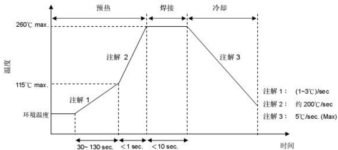
波峰焊曲线
