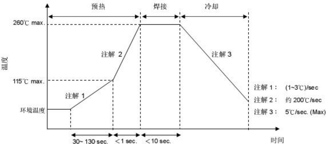
波峰焊曲线
